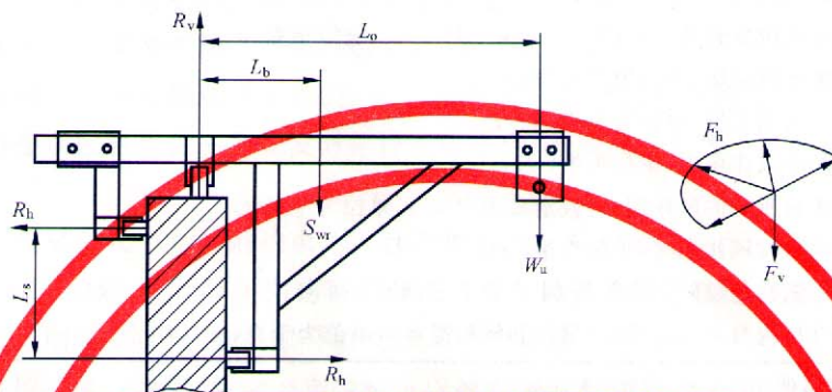
图 11 女儿墙卡钳
