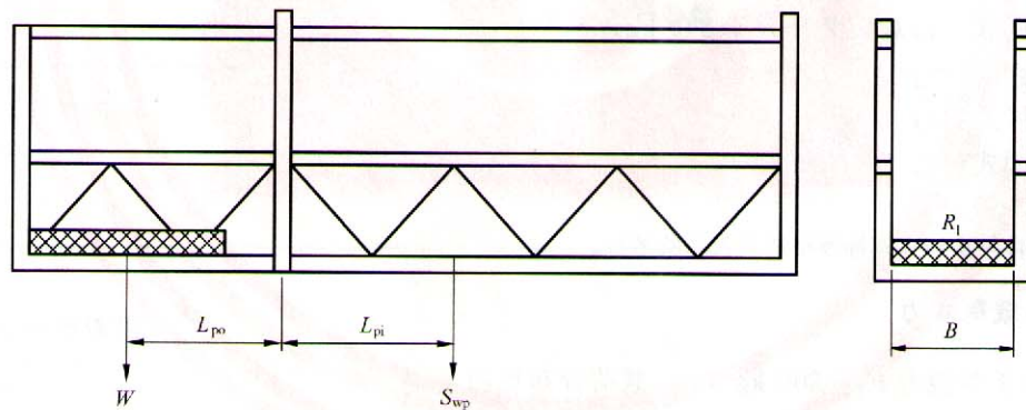
图 6 悬臂平台
