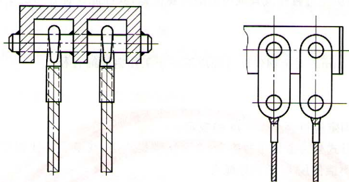
图 16 典型悬挂点示例
